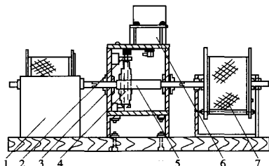
图 T0207-1 耐崩解性试验仪
