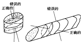
图 T0225-3 对各向异性岩施加荷载的正确方向
